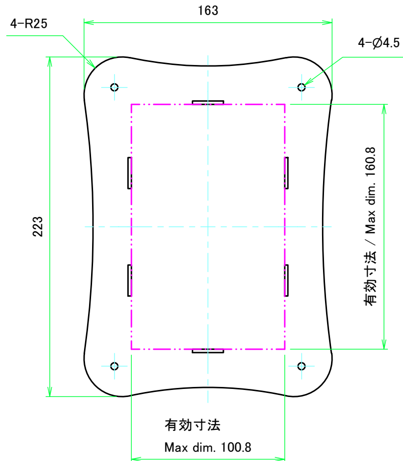
上カバー表面 / Top cover Frontside
